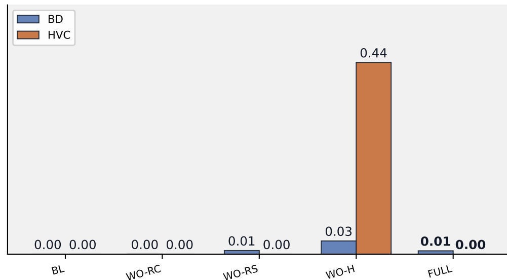
BD / HVC ↓
